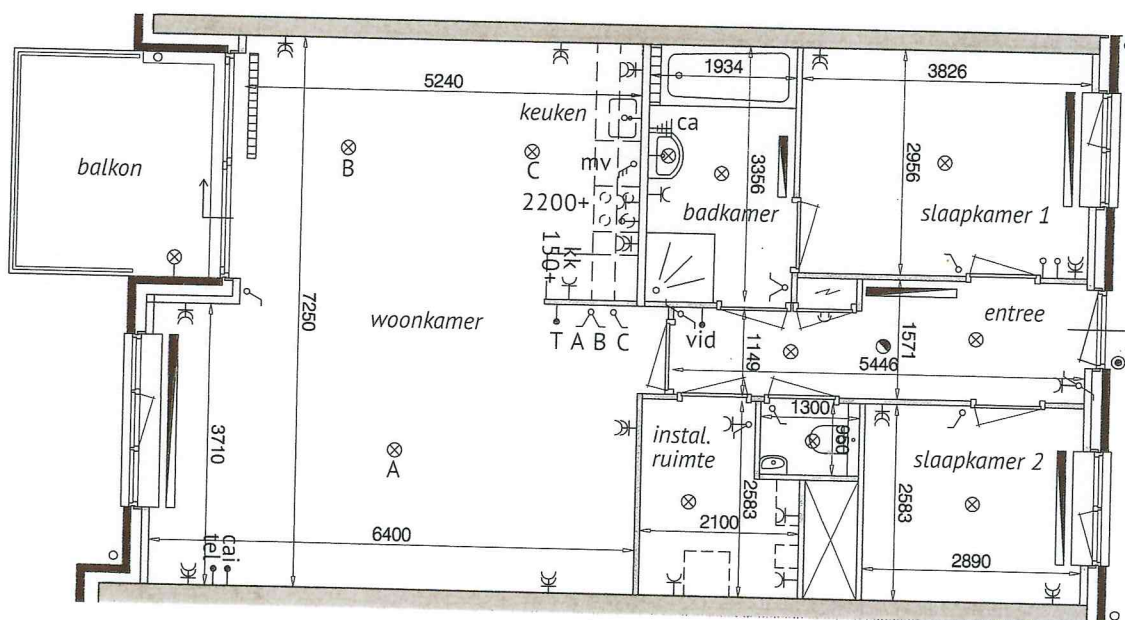
Woningtype B1 - Bouwnummers 3 & 12
